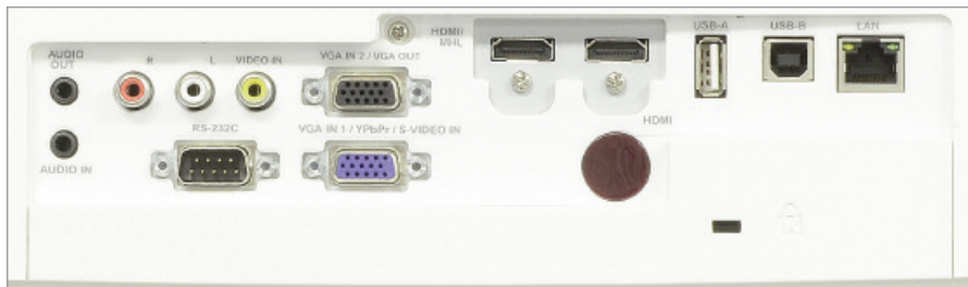
EK-305U • WUXGA • 3LCD projector.
